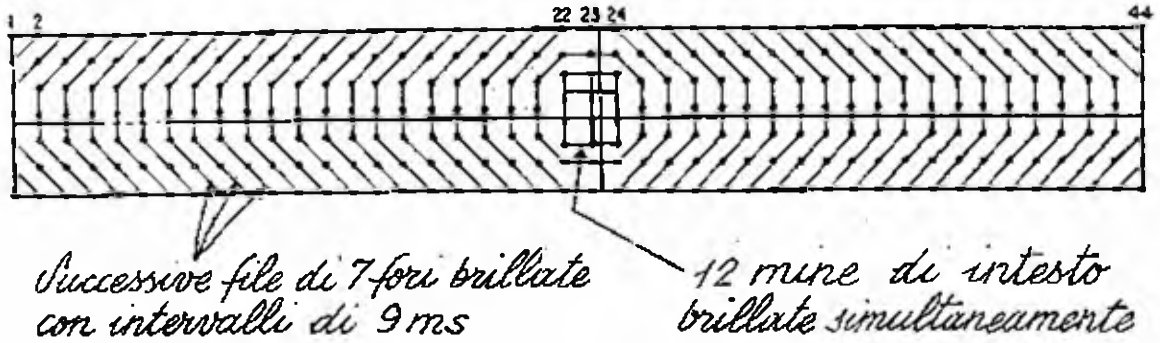
Fig. 16.10 - Miniera di Star Lake: schema della volata (Du Pont)
