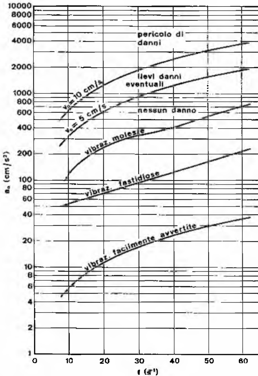
Fig. 15.16 - Curve di uguale effetto fisiologico sulle persone (secondo Reichert e Meister) e di uguale effetto dannoso sugli edifici secondo il criterio delle velocità ( a_0 sta per a_{max} e v_0 sta per v_{max} del resto)
