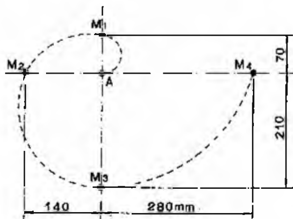
Fig. 6.17 - Intesto a spirale nella miniera di Montepuni (Cagliari), della Soc. Montepuni e Montevecchio
