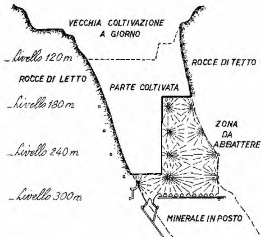
Fig. 16.37 - Schema della volata di 16 700 mine fatta brillare nella miniera Frood-Stobie (Ontario), della International Nickel Company
