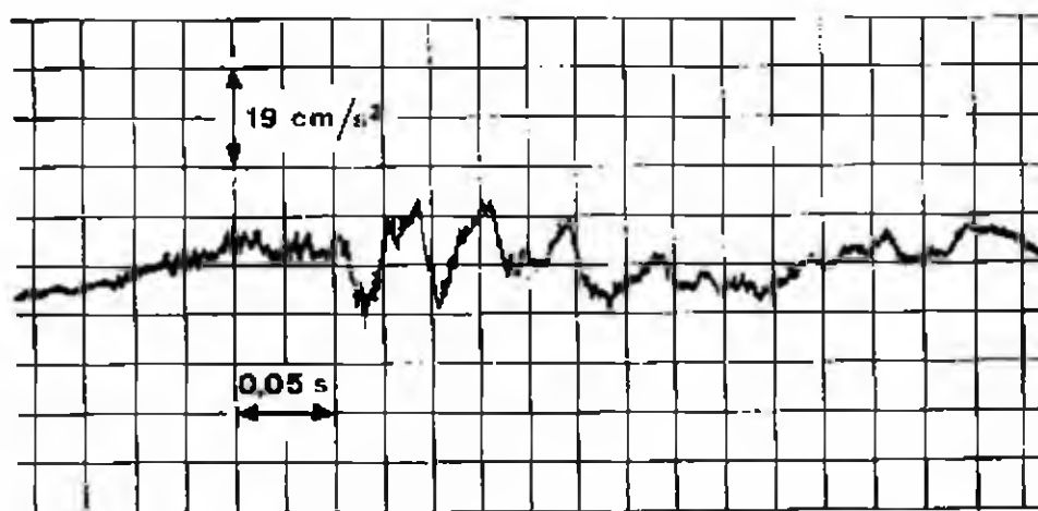
Fig. 15.2 - Sismogramma relativo ad una esplosione in cava di pietrisco, rilevato a distanza di circa 400 m dal punto di scoppio; se ne ricavano i valori: a_{\text{max}} = 11 \text{ cm/s}^2 f = 25 \text{ cicli/s}
