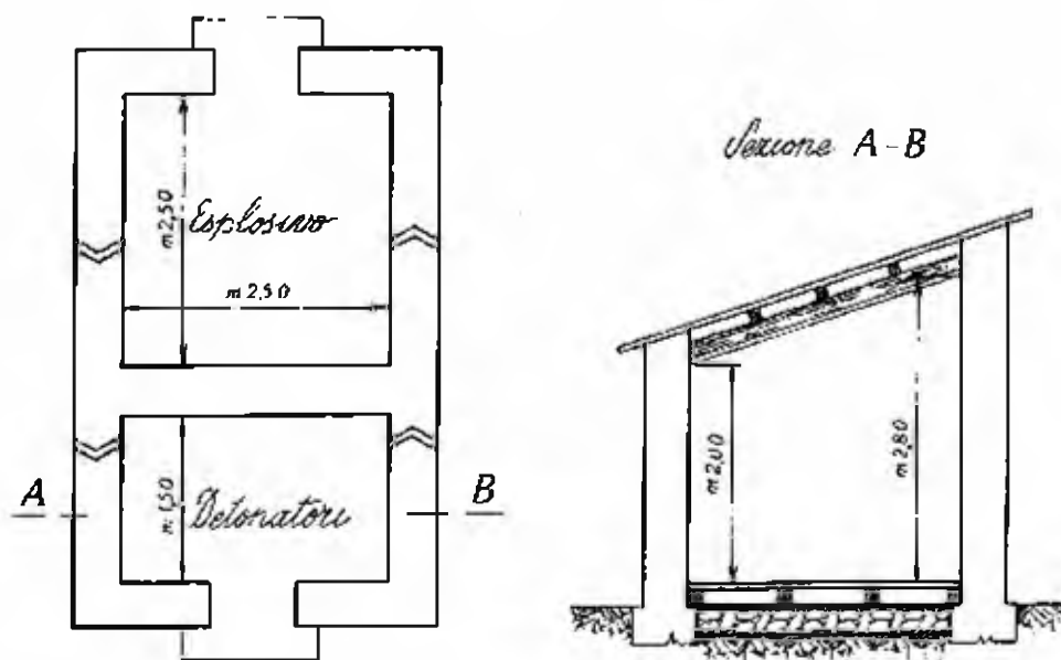
Fig. 7.6 — Casotto in muratura per 200 kg di esplosivo di 2ª categoria (non sono indicati il recinto e la gabbia di Faraday)
