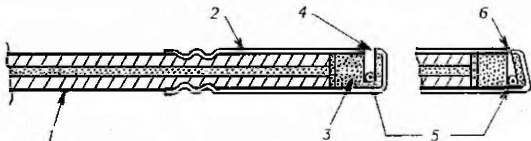
Fig. 10.12 - Connettore per spittercord: 1) miccia da accendere; 2) bossolo del connettore; 3) carica esplosiva; 4) fessura aperta; 5) spittercord; 6) fessura chiusa (Coast Manuf. and Supply Co.)
