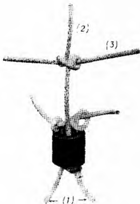
Fig. 8.55 - Scatola di raccordo per derivazione di più micce detonanti: (1) = micce derivate; (2) spezzone di miccia; (3) = miccia maestra (Insign-Bickford Co.)
