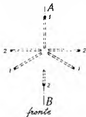
Fig. 6.4 - Intesto a forbice costituito da due terne di mine a piramide in parte intrecciate: a sinistra, fronte; a destra, profilo
