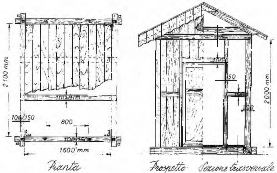
Fig. 7.7 — Casotto di legno per 500 kg di esplosivo di seconda categoria (ripreso dal Regolamento di pubblica sicurezza)
