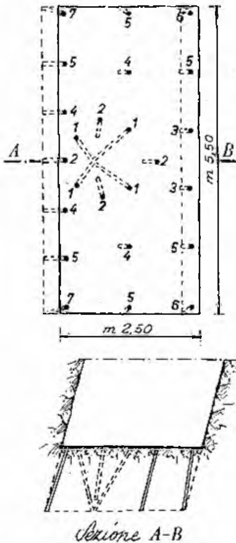
Fig. 16.40 - Schema di volata per pozzo rettangolare inclinato
