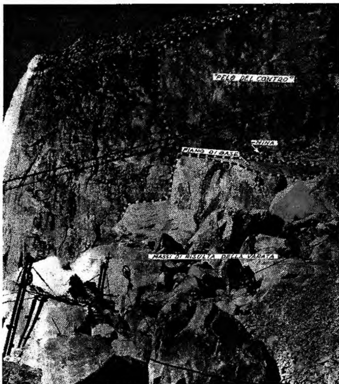
Fig. 13.42 - Varata con taglio di base e piccola mina a camera nella cava di marmo « Campanili » (Carrara), Ditta Adolfo Corsi e Soc. Montecatini (foto I. Bessi, Carrara)
