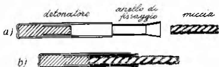
Fig. 8.14 - Tubicino Kinsmen per sostituire l'arriccatura del detonatore intorno alla miccia: a) componenti; b) accoppiamento eseguito
