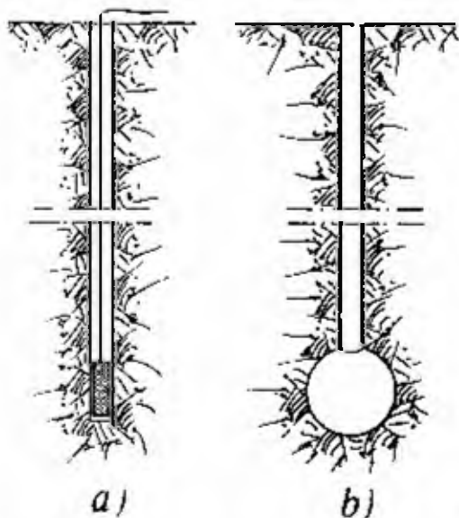
Fig. 13.40 - Preparazione della cavità per una mina a fondo allargato: a) prima carica; b) cavità finale ottenuta
