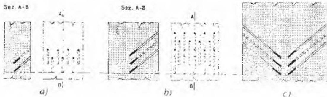
Fig. 17.23 - Demolizione di un muro con file di mine laterali: a) con due file di mine; b) con tre file di mine; c) con tre file di mine da ambo i lati
