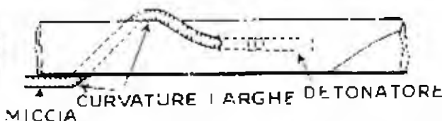
Fig. 8.20 - Innesco laterale interno con miccia a larga spirale (Coast Manuf. and Supply Co.)
