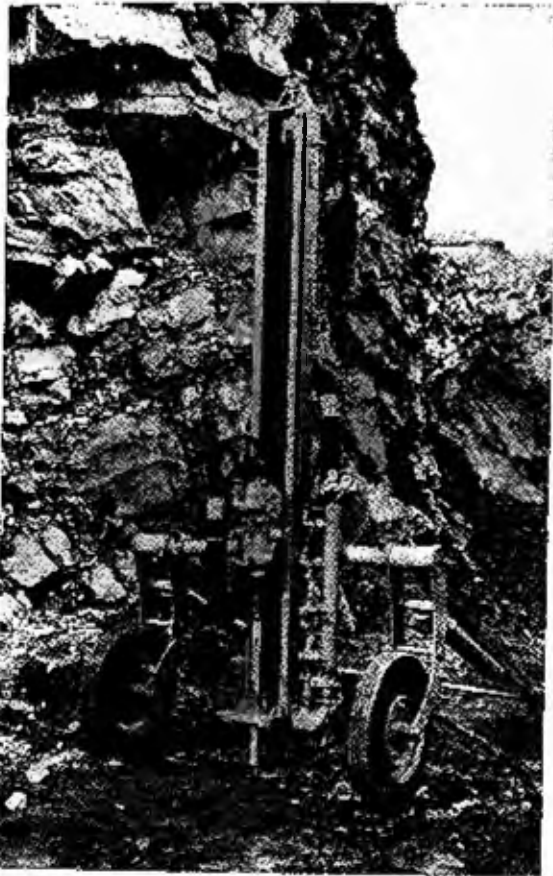
Fig. 5.10 - Perforatrice penetrante Stenuick tipo BB-AS pronta per iniziare un foro verticale (ing. G. Radaelli, Milano; foto Photographie Industrielle, S.P.R.L. Bouters, Bruxelles)
