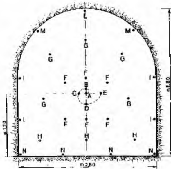
Fig. 16.27 - Volata con intesto a spirale nelle miniere di Monteponi (Cagliari), della Soc. Monteponi e Monteverchio.
