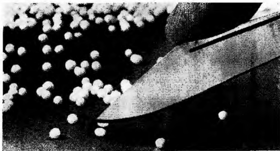
Fig. 3.5 - Granuli sferoidali (prilli) di NA ottenuti con la caduta di soluzione di NA da una torre (Gulf Oil Corporation, Chemicals Department)
