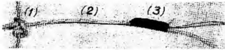
Fig. 11.21 - Miccia detonante innescata con uno spezzone: 1) collegamento dello spezzone alla miccia maestra; 2) spezzone; 3) innescamento dello spezzone (Ensign Bickford Co.)
