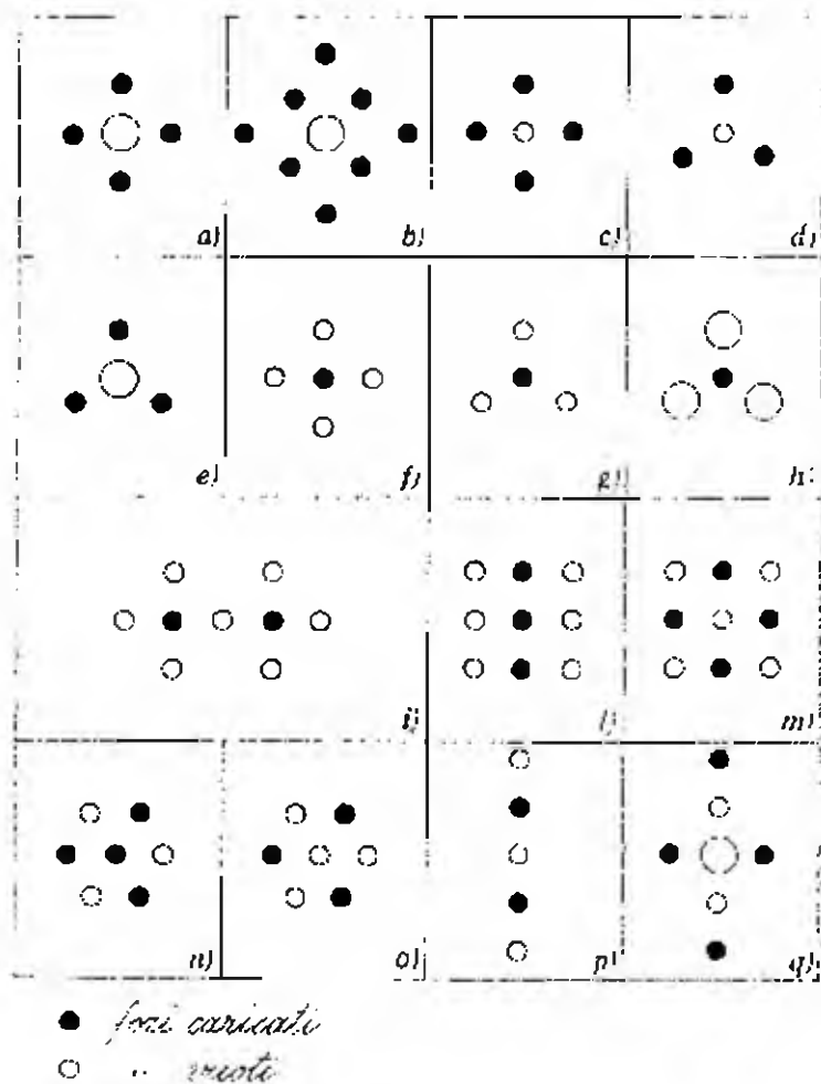
Fig. 6.9 - Tipi di intesto con mine parallele (burn cut): a) e b) intesto Michigan; i rimanenti sono intesti di tipo canadese: c) d), e), a quadrifoglio; f), g) h), i), a quadrifoglio rovesciato; l), m), intesto quadrato; n) o), intesto esagonale; p), q), intesto a fessura
