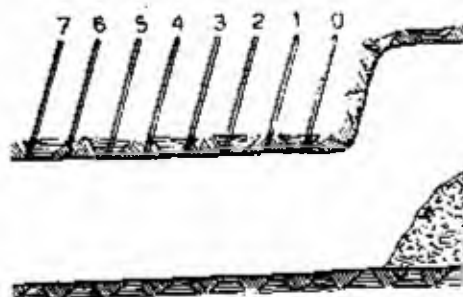
Fig. 16.33 (a sinistra) - Volata per cantiere alto, con sottogiallo
