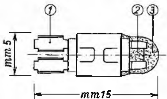
Fig. 9.1 - Testina di accensione: 1) lamine di attacco dei reofori; 2) resistenza elettrica; 3) miscela di accensione (Montecatini Edison)
