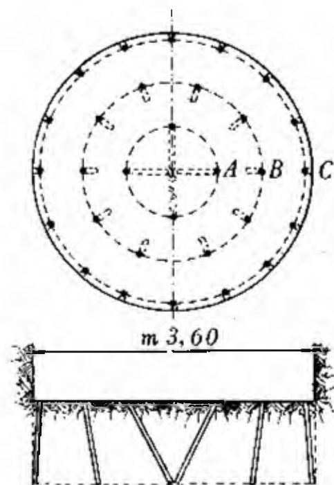
Fig. 16.42 - Schema di volata per pozzo circolare verticale
