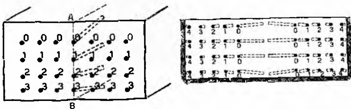
Fig. 16.12 - Sbanco con mine orizzontali: a sinistra con mine a ventaglio; a destra con mine a V
