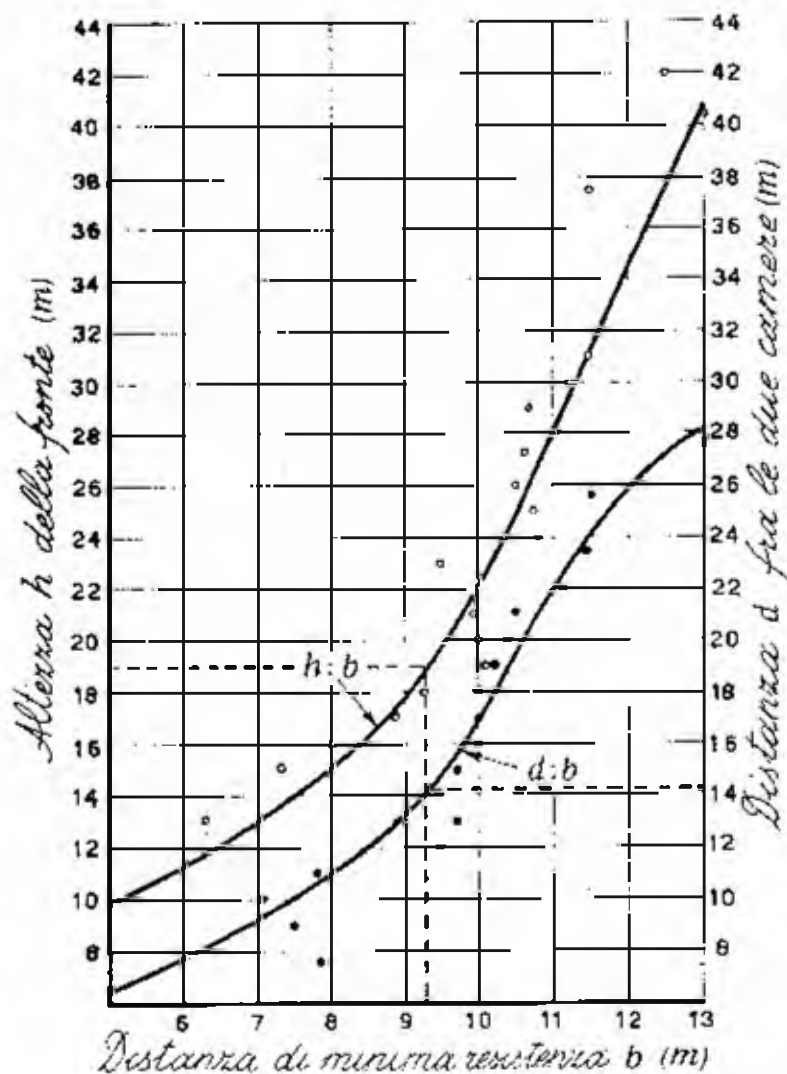
Fig. 14.5 - Rapporto tra l'altezza della fronte e la distanza di minima resistenza nonché rapporto fra la distanza delle due camere e la distanza di minima resistenza (No. 62 Hefte)
