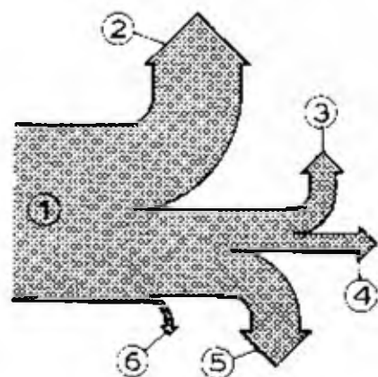
Fig. 15.1 - Ripartizione dell'energia sviluppata dall'esplosione di una carica: 1) carica iniziale; 2) perdita a massiccio; 3) perdita all'atmosfera; 4) parte che causa proiezione dell'abbattuto; 5) parte che causa frammentazione dell'abbattuto; 6) parte che causa il distacco della parte abbattuta da quella che rimane in posto
