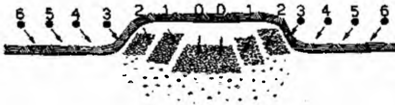
Fig. 16.1 - Frantumazione per urto fra i detriti lanciati da mine successive in una volata con ritardi di millisecondi (Du Pont)
