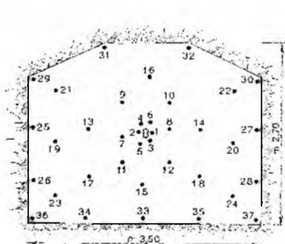
Fig. 6.14 - Una volata completa con inteso Coromant (schiuma Atlas Copco)
