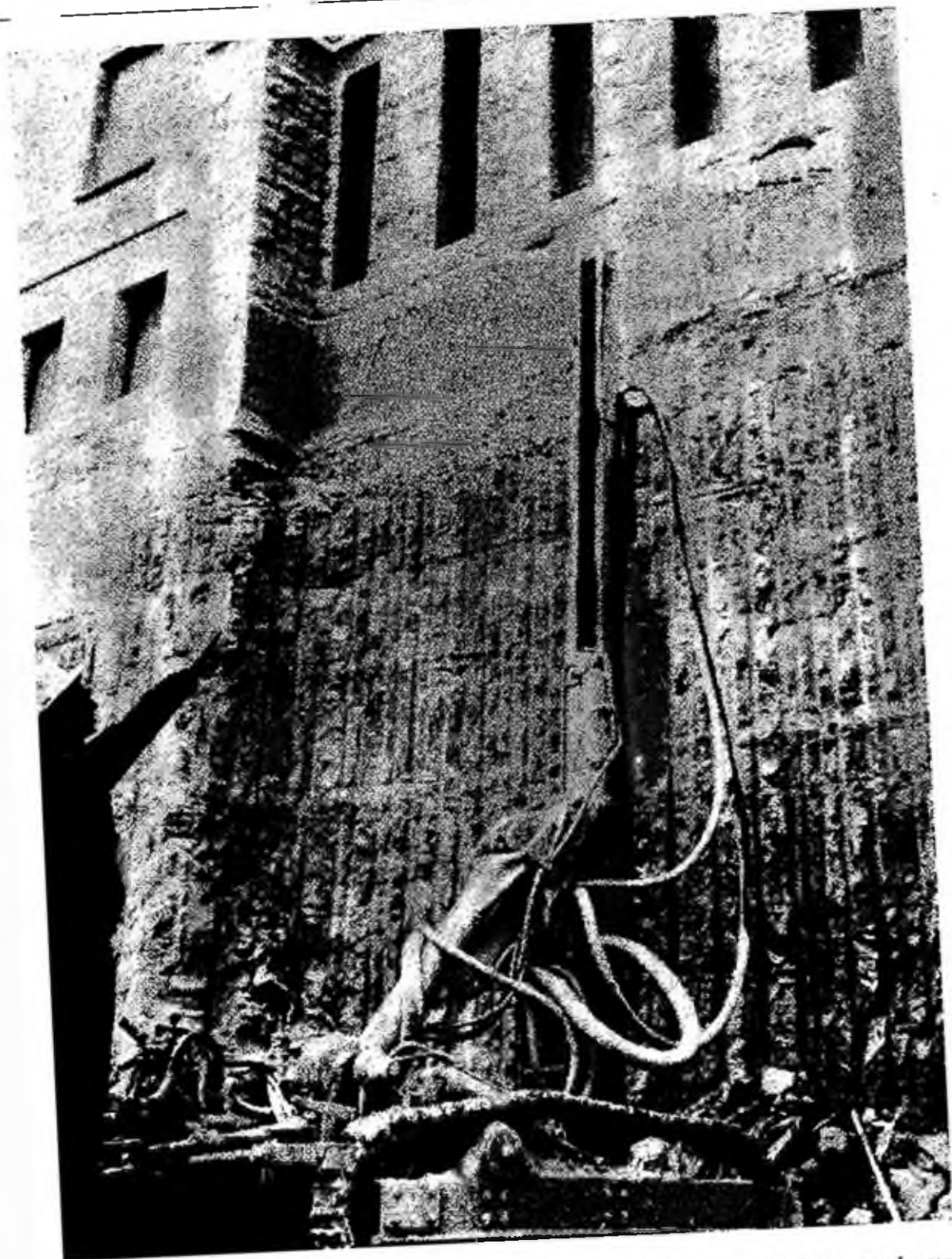
Fig. 13.18 - Sbancamento effettuato a ridosso di una costruzione, con il tiro a cuscinetto (Blasters' Handbook, 15 a ed., 1966, Du Pont)
