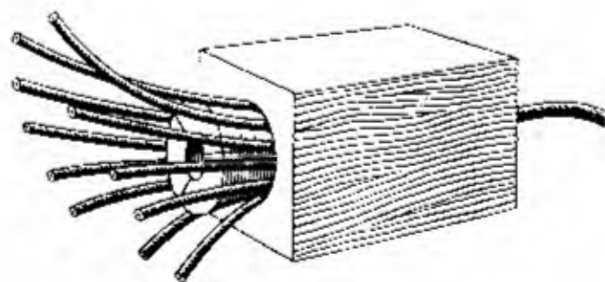
Fig. 10.11 - Scatola raccordo per l'accensione di più micce a lenta combustione (Manuel Bickford, 3ª ed., 1961, Stab. Bickford, Roma)
