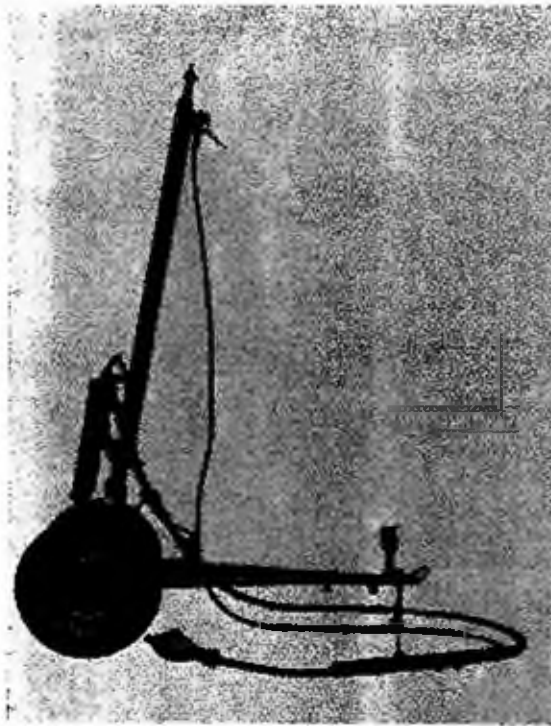
Fig. 5.4 (a sinistra) - Sbancatore per perforatrici pesanti fino a 30 kg, impiegabile con aste estensibili per profondità fino a 10 m (Atlas Copco; servizi fotografici Costa, Milano)
