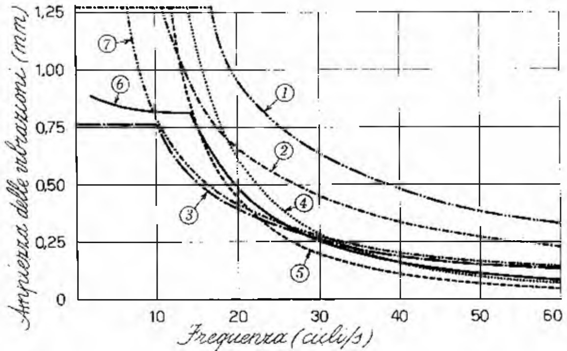
Fig. 15.4 - Zone di sicurezza e di danni nel diagramma: ampiezza delle vibrazioni-frequenza
