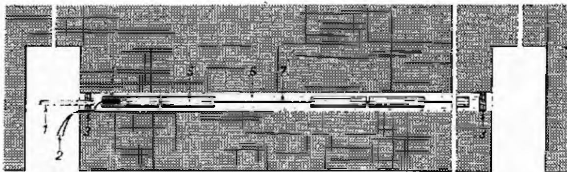
Fig. 18.12 - Abbattimento del carbone con fori lunghi laterali e con acqua in pressione. Planimetria: 1 = tubo di adduzione dell'acqua compressa; 2 = rofori dell'innescò; 3 = tappi di tenuta; 4 = innescò; 5 = cartuccia della carica; 6 = acqua in pressione; 7 = miccia detonante (Blasting Practice, 3 a ed., 1962, Imp. Chem. Industries)
