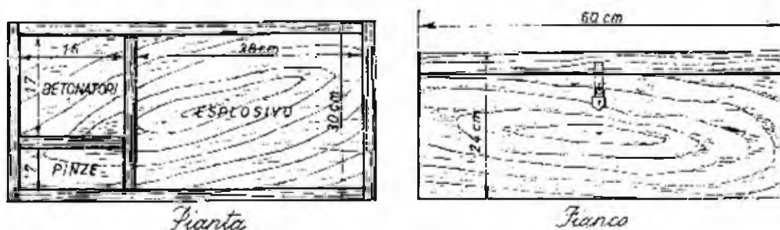
Fig. 7.13 - Cassette di legno per il deposito di esplosivo in cantiere durante il turno di lavoro
