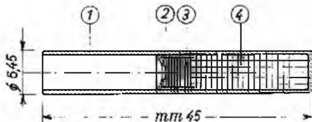
Fig. 8.3 - Detonatore per miccia: 1 = bossoletto in alluminio; 2 = opercolo in alluminio; 3 = carica primaria di azostifnato di piombo; 4 = carica secondaria di pentite (Montecatini Edison)
