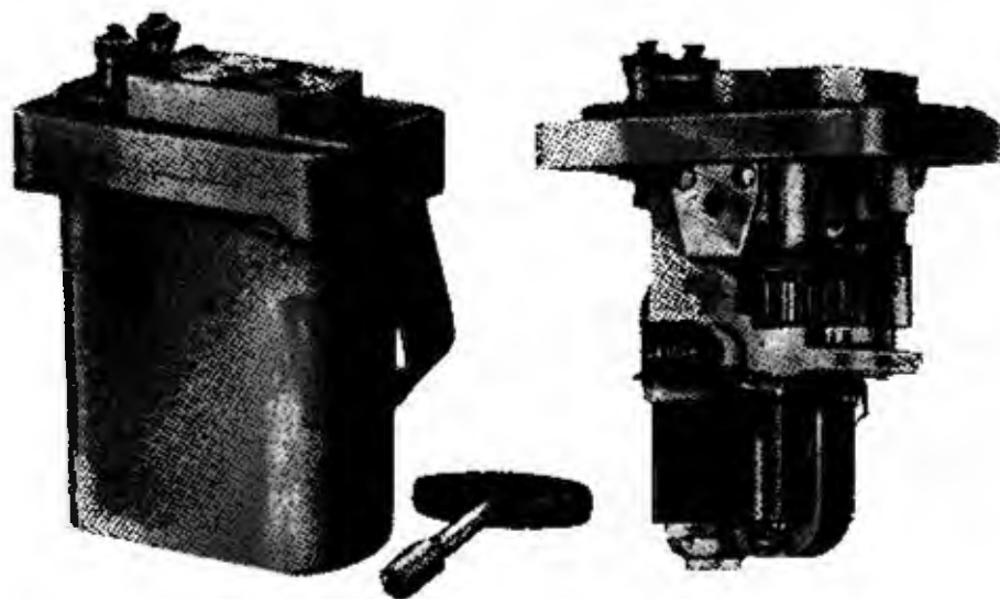
Fig. 11.5 - Esploditore Schaffler tipo 750 con azionamento a molla, per 200 detonatori in serie con reofori di rame lunghi 2 m: a sinistra, chiuso; a destra, senza scatola
