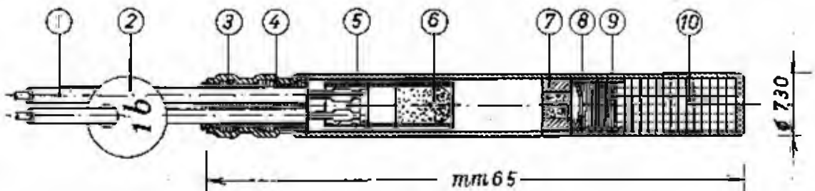
Fig. 9.3 - Innesco a ritardo: 1) filo di rame viplato; 2) medaglietta con l'indicazione del tempo di ritardo; 3) tappo di gomma; 4) bossolotto in alluminio; 5) guaina di protezione; 6) testina di accensione; 7) tubo di ritardo; 8) opercolo in alluminio; 9) carica primaria di azostifnato di piombo; 10) carica secondaria di pentrite (Montecatini Edison)
