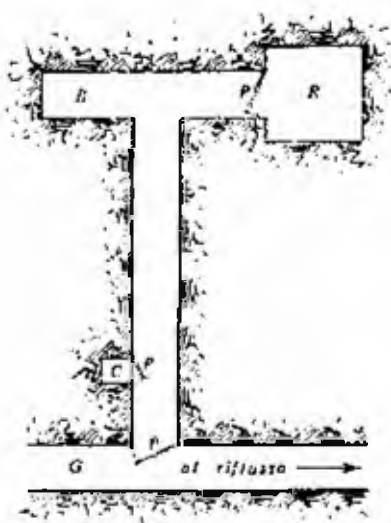
Fig. 7.10 (a sinistra) - Riserverta per meno di 50 kg di esplosivo: R = riserverta, C = nicchia per detonatori, E = nicchia per l'esplosivo, P = porta, G = galleria al riflusso
