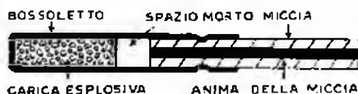
Fig. 8.6 - Miccia introdotta scarsamente nel detonatore lasciando uno spazio morto (Coast Manuf. and Supply Co.)
