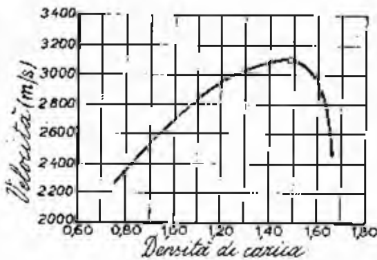
Fig. 2.9 - Relazione fra la densità di carica e la velocità di detonazione per un esplosivo di tipo cheddite
