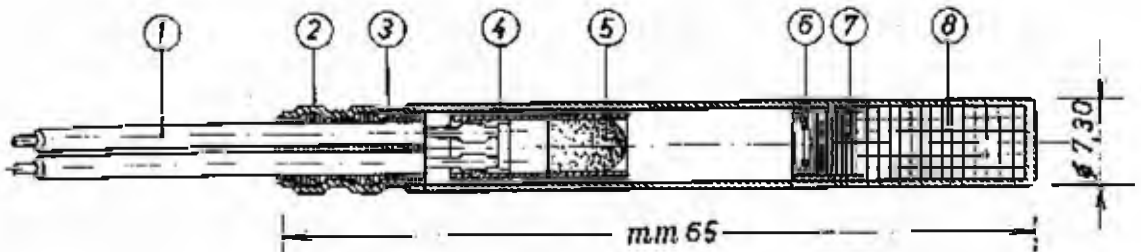
Fig. 9.2 - Innesco istantaneo: 1) filo di rame viplato; 2) tappo in gomma; 3) bossolotto in alluminio; 4) guaina di protezione; 5) testina di accensione; 6) opercolo in alluminio; 7) carica primaria di azostifnato di piombo; 8) carica secondaria di pentrite (Montecatini Edison)
