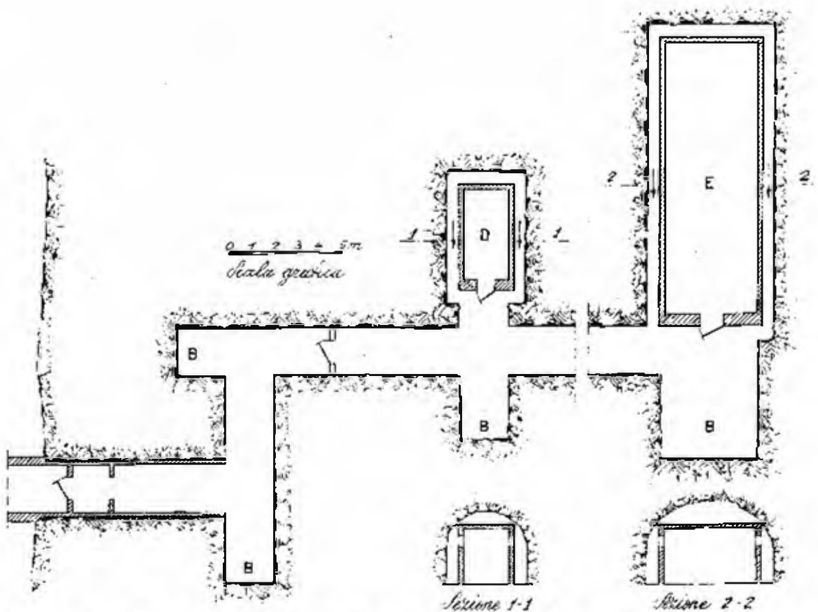
Fig. 7.9 - Tipo di deposito permanente sotterraneo per 8 000 kg di esplosivo di 2° categoria e per 50 000 detonatori; E = cancri dell'esplosivo; D = locale per i detonatori; B = nicchioni ammortizzatori
