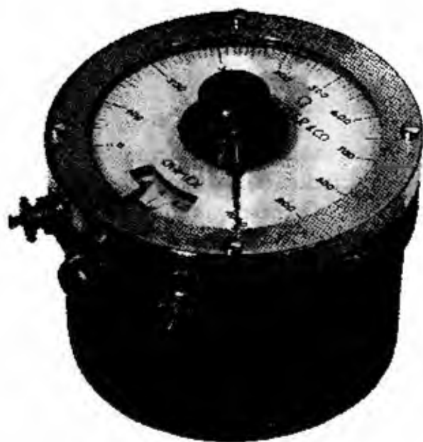
Fig. 11.8 - Prova esplositori tipo Ohmex (Schaffner)
