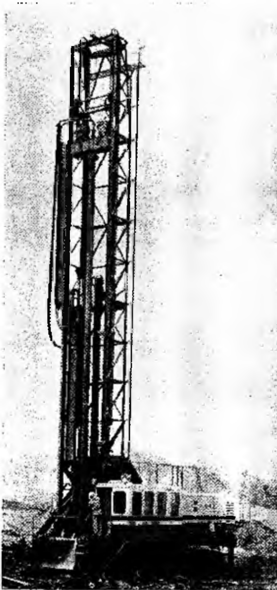
Fig. 5.7 - Super wagon drill Bucyrus - Eric, 61-R pesante 74 t, per fori di diametro 37 ÷ 46 cm, in azione nella Sinclair Mine (Kentucky) della Peabody Coal Co.
