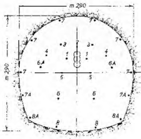
Fig. 6.15 - Intesto di tipo super cut
