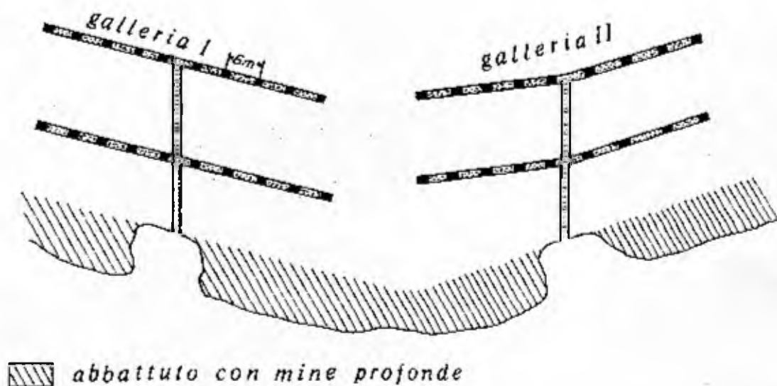
Fig. 13.36 - Grande mina con 38 camere in due gallerie, ognuna con due traverse, a Puerto Cabello, Venezuela (Nobel Hefte)
