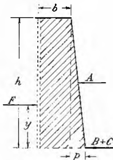
Fig. 14.11 - Forze in gioco nell'azione di una mina profonda verticale con fronte di abbattimento inclinato (L'Industria Mineraria)
