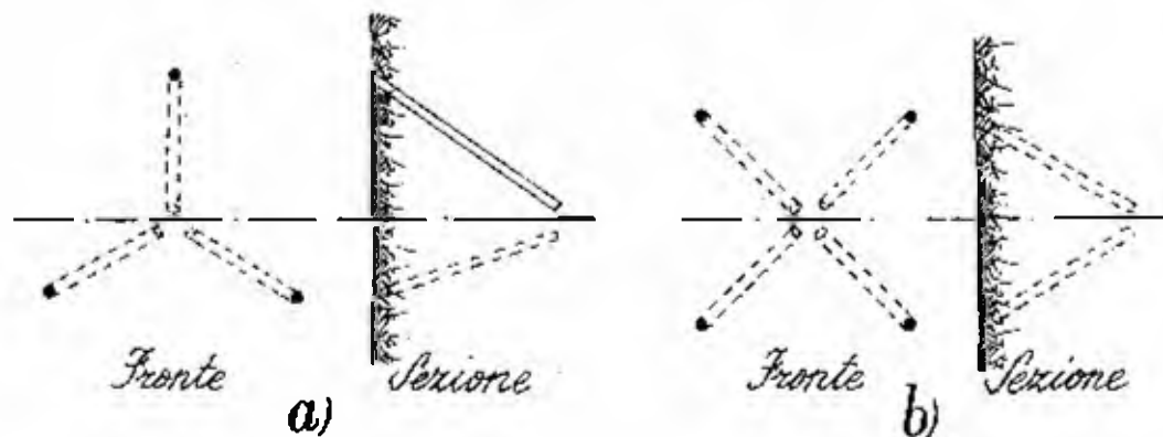
Fig. 6.2 - Intesto a piramide: a) con tre mine b) con quattro mine
