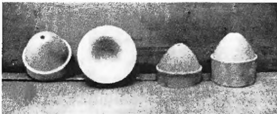
Fig. 17.39 - Cariche cave per pctardaggio, della Ditta Mangiarotti, Codroipo (Udine)
