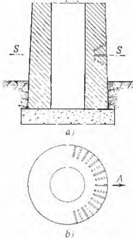
Fig. 17.31 Demolizione di una ciminiera: a) sezione verticale; b) sezione orizzontale all'altezza del piano SS; A = senso di caduta dell'opera (Revue de l'Industrie Minière)
