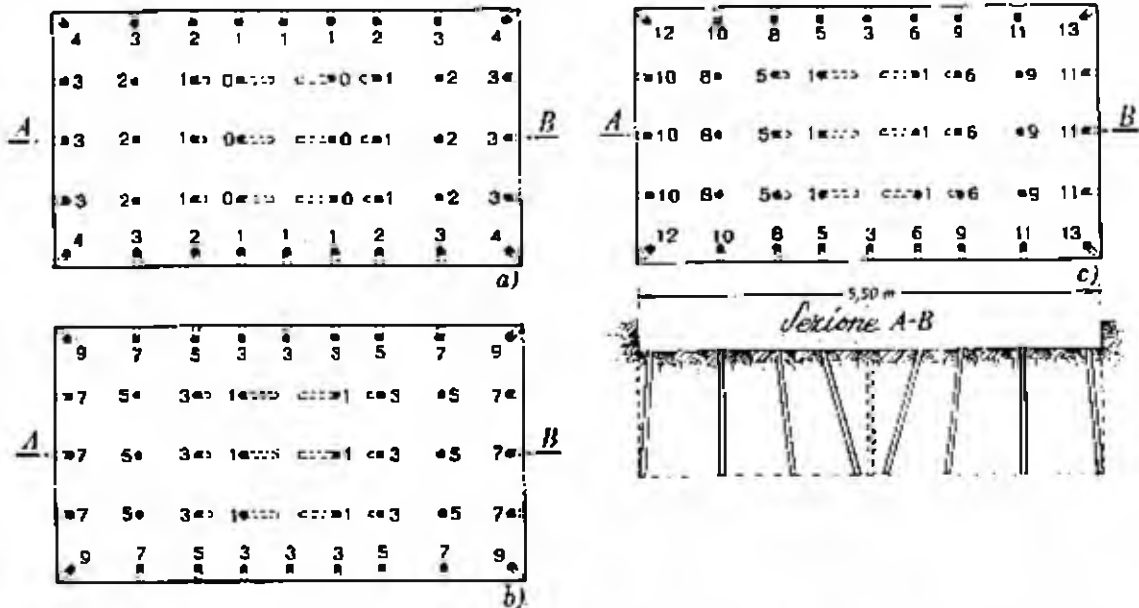
Fig. 16.39 - Schemi di volate per pozzo rettangolare verticale: a) per ottenere cumulo di abbattuto piramidale; b) idem; c) per ottenere cumulo piatto
