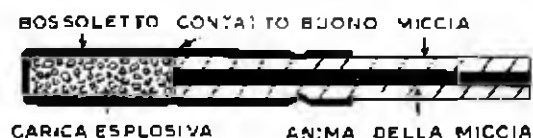
Fig. 8.5 - Miccia tagliata bene e inserita bene nel detonatore (Coast Manuf. and Supply Co.)
