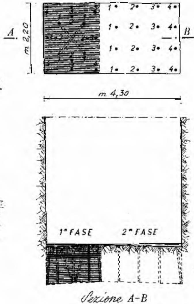
Fig. 16.41 - Schema di volata per approfondimento in due tempi di un pozzo rettangolare
