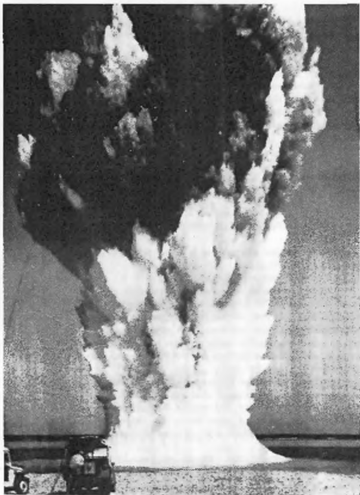
Fig. 17.1 Btillamento in mare di 1 000 kg di esplosivo per sismica a rifrazione, nella zona di Dungenan, nel Sudan (Ente Nazionale Idrocarburi, ENI);
