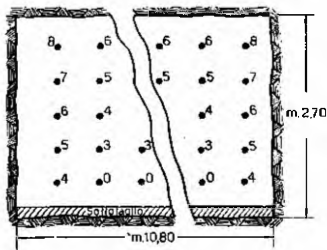
Fig. 16.34 (sopra) - Volata per coltivazione a gradino rovescio
